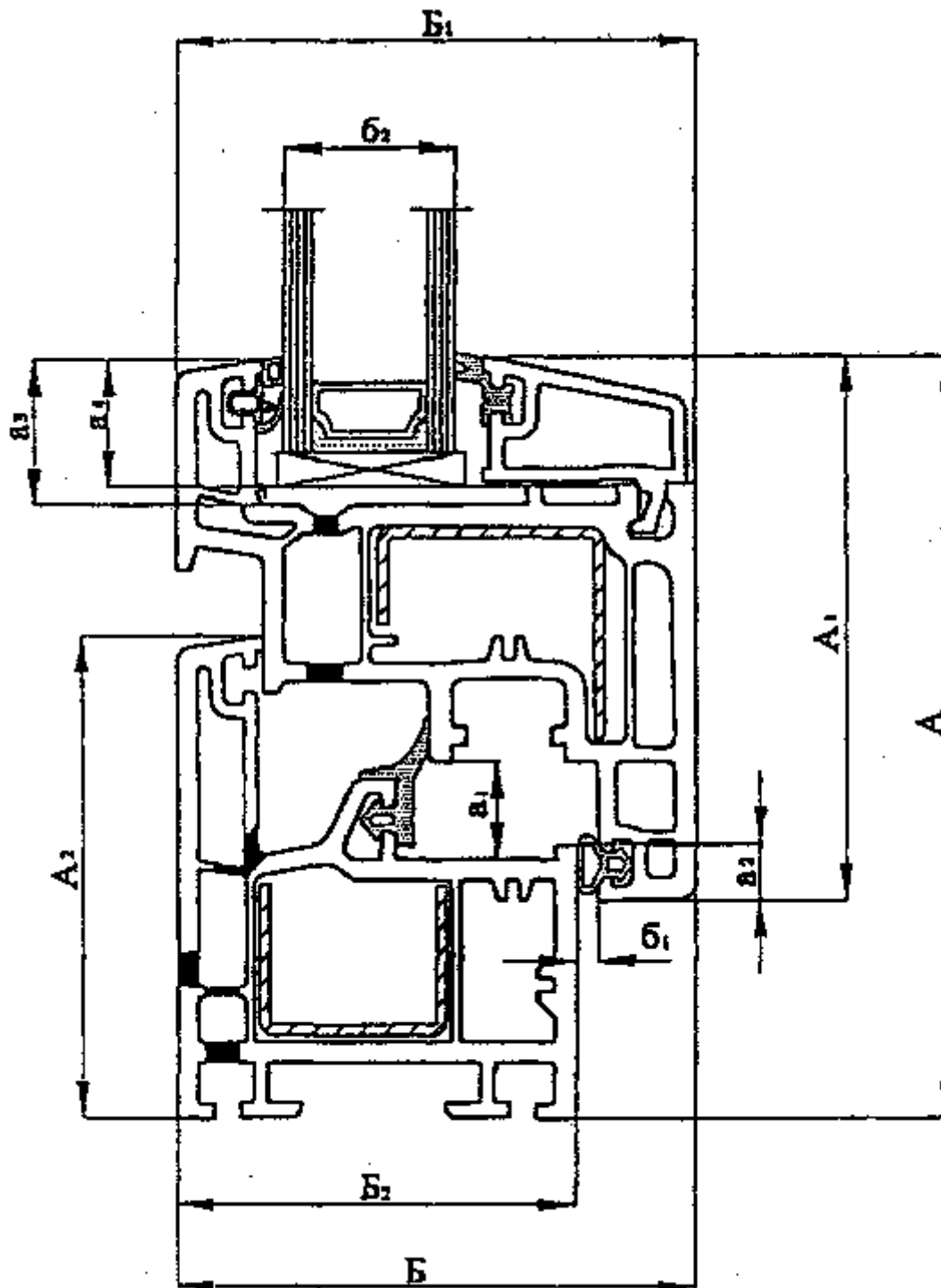
Рисунок А.1 - Основные детали комбинации профилей
