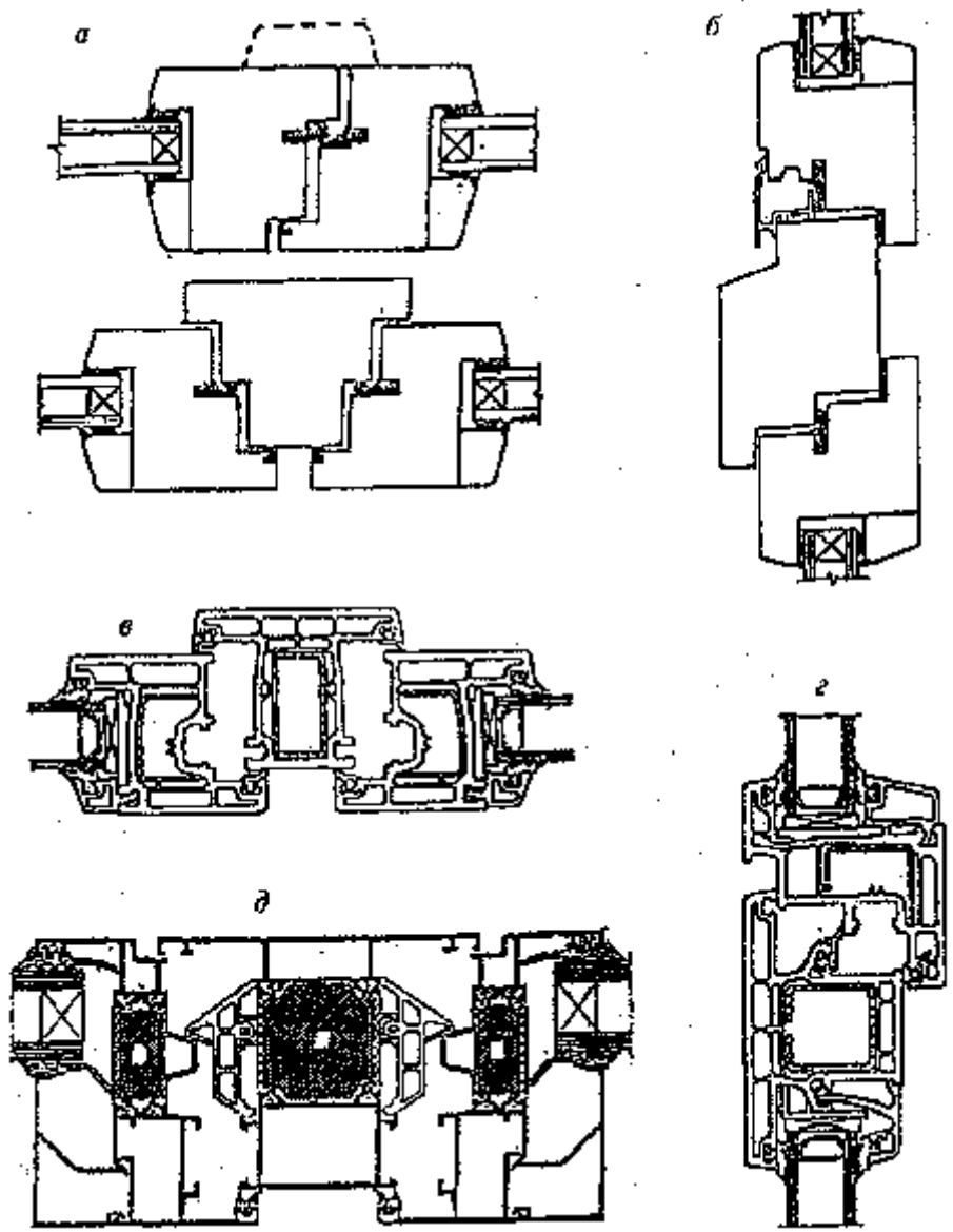
а - вертикальные безимпостный (ппультровой) и импостный притворы деревянного оконного блока; б- горизонтальный импостый притаор деревянного оконного блока; в - импостный притвор оконного блока из ПВХ профилей; г - узел импостного соединения открывающейся створки и остекленной коробки; д - импостный притвор оконного блока из алюминиевого сплава
