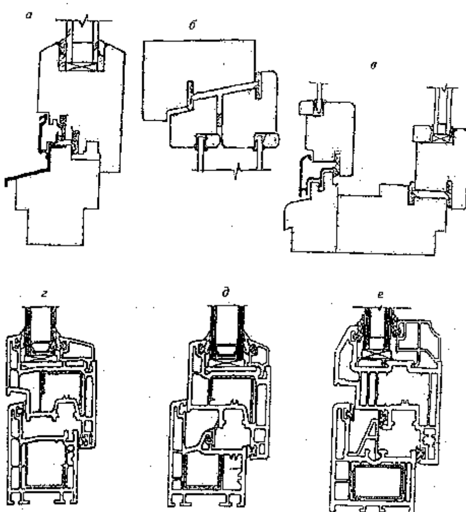
а - конструкция с двумя средними уплотнениями; б - конструкция со средним и внутренним уплотнениями; в - конструкция с двумя средними и внутренним уплотнениями; г - конструкция с наружным и внутренним уплотнениями; д - конструкция со средним и внутренним уплотнениями; е - конструкция с наружным, средним и внутренним уплотнениями
